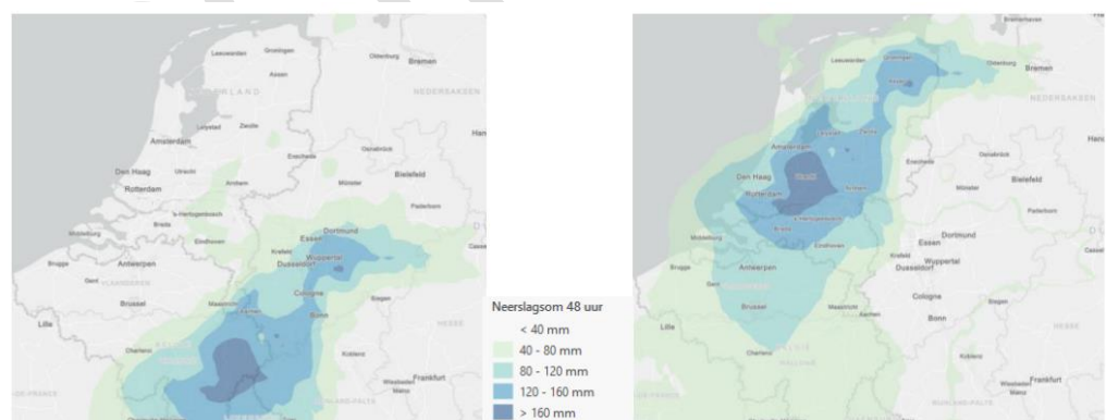
Figuur 4: 48-uur neerslagsom juli 2021; werkelijke situatie (links) en een voorbeeld van een verschoven situatie (rechts); uit: Deltares, 2022
