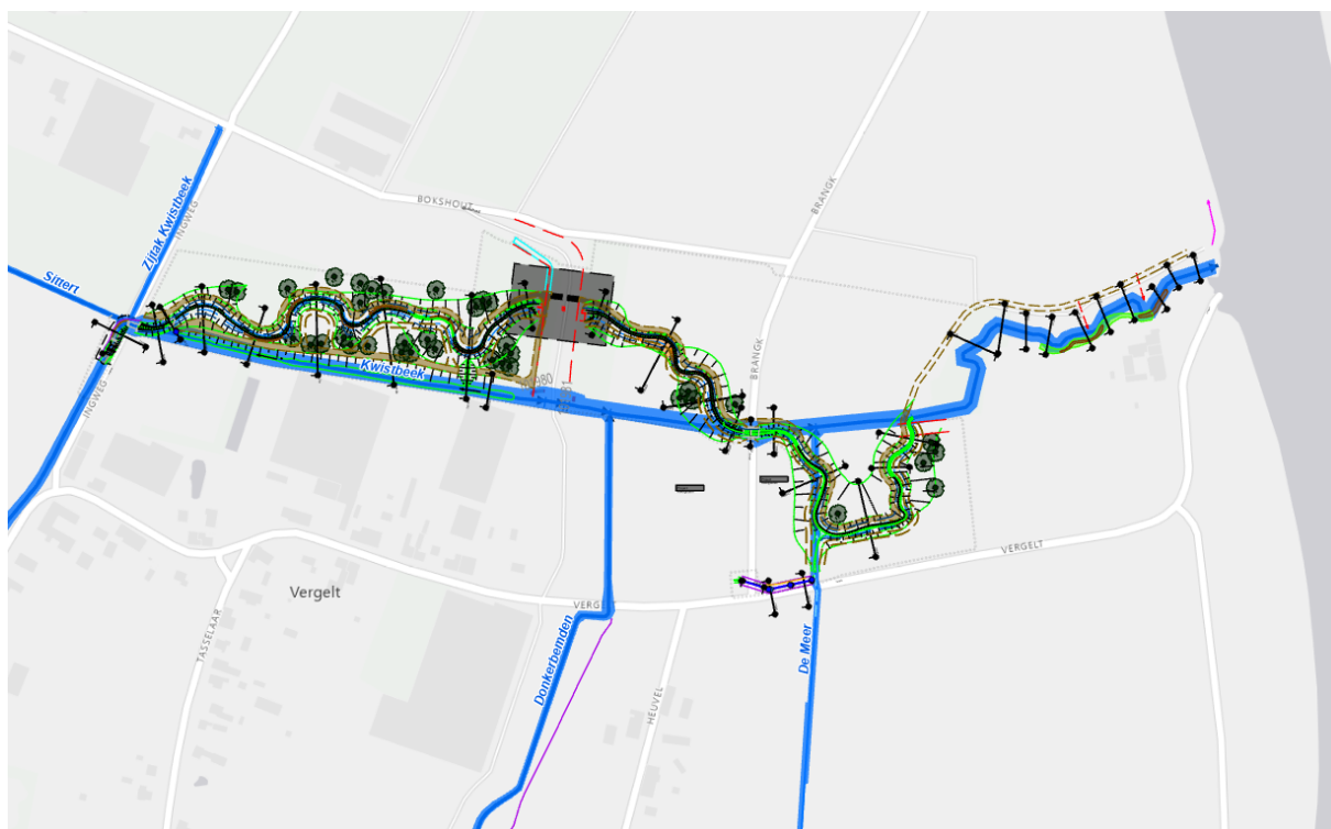
Figuur 1 Overzicht projectgebied Kwistbeek met de DO tekeningen en de bestaande werkingsgebieden van Waterschap Limburg als achtergrond.
